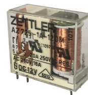
Relè 6V SPST - AZ725-1C-6DM - ZETTLER 6VDC 16A 250VAC Numero di PIN: 8 Dimensioni (mm): 25.5 x 29.5 x 13
