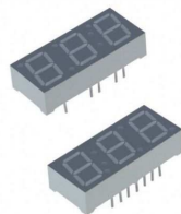
Display LED verde triplo BT-M402RI Caratteristiche Display LED verde triplo P/N: BT-M402RI Connessione: Anodo comune multiplex Dimensioni: 30x16x7mm
